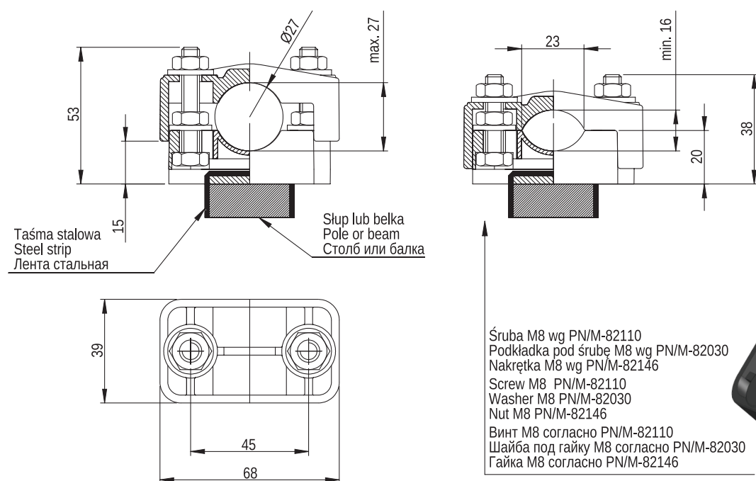
Obejma kablowa KO 27 T
