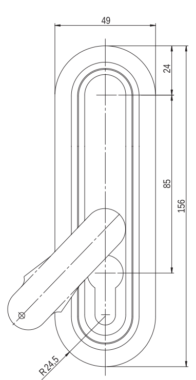
Zamek HS 01 MATERIAL: Korpus - PA 6 GF30; kolor czarny, biały, szary wg RAL.
