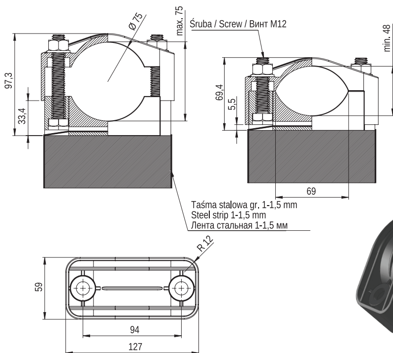
Obejma kablowa KO 75 TP
