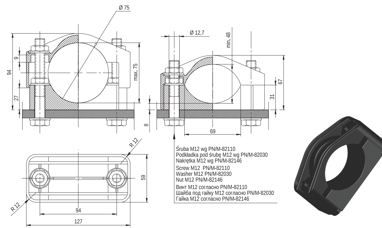
Obejma kablowa KO 75
