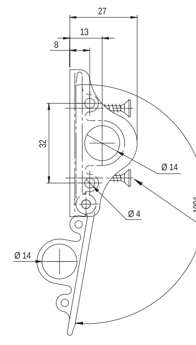
Escutcheon for 'E z ' Lock
