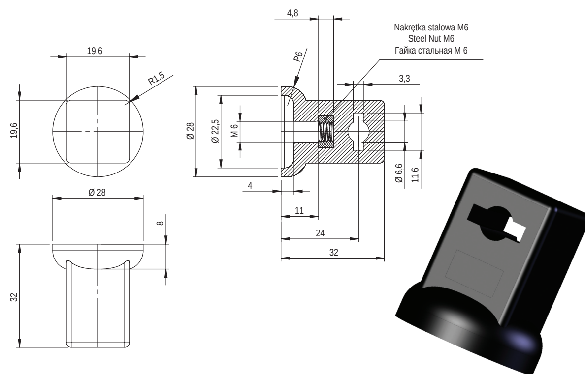
Prowadnica Ø 6 PR6/2
