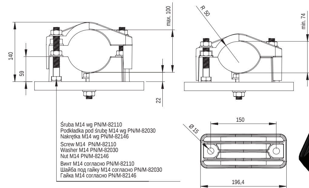
Obejma kablowa KO 100 OTW
