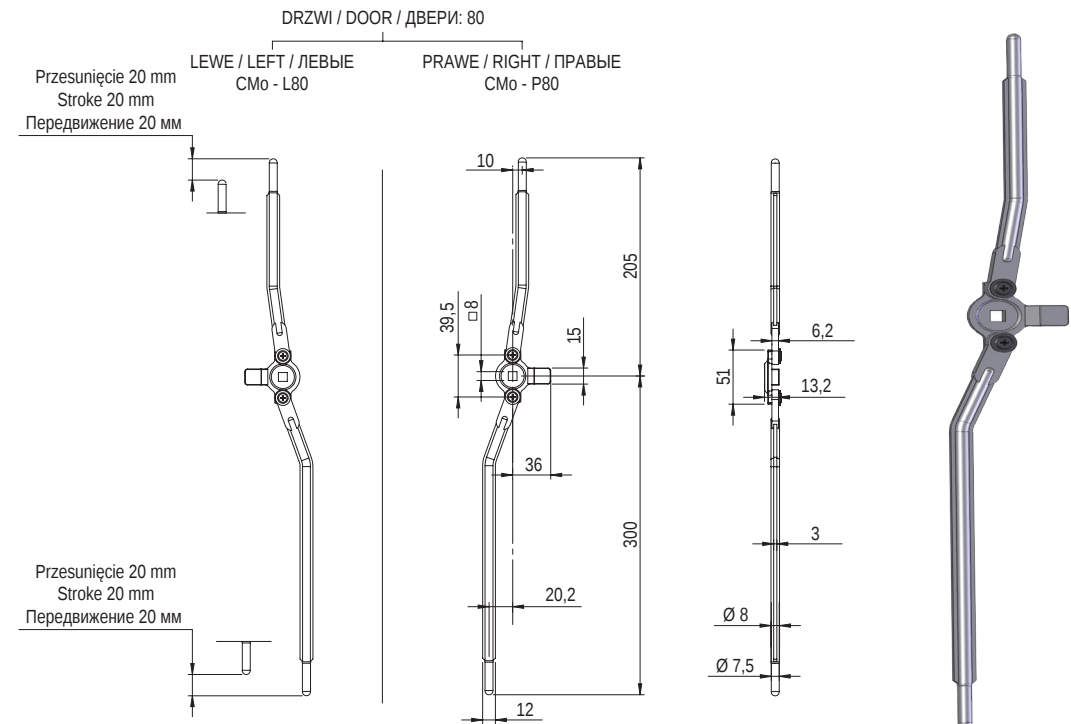
Cięgna z mechanizmem obrotowym Cmo - P, L 50
