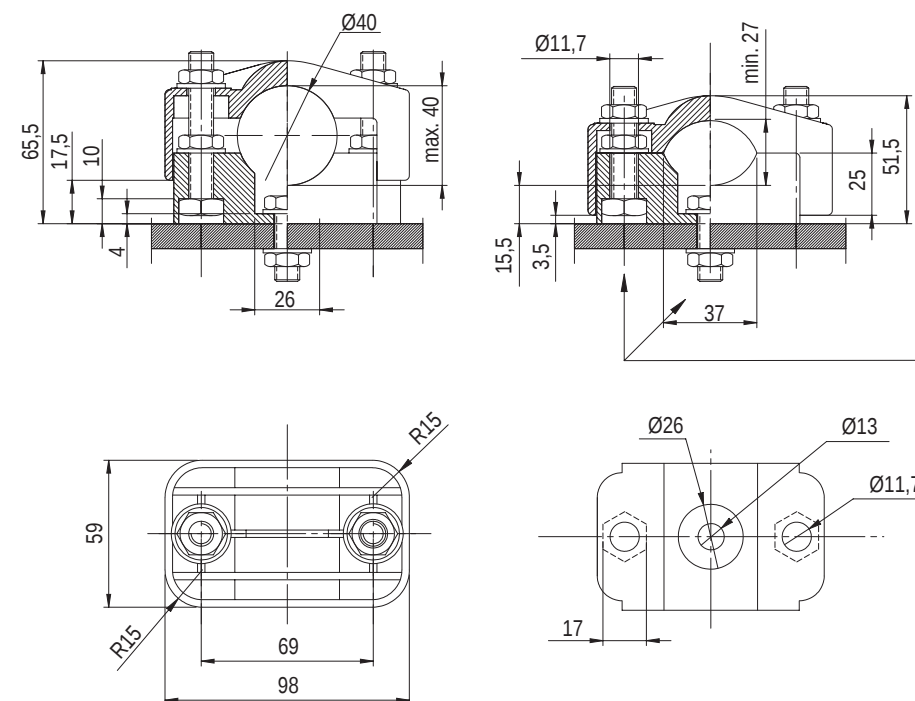
Obejma kablowa KO 40 OTW
