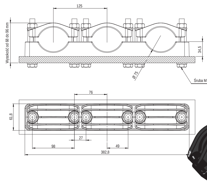
Obejma kablowa zespolona KO 75/3
