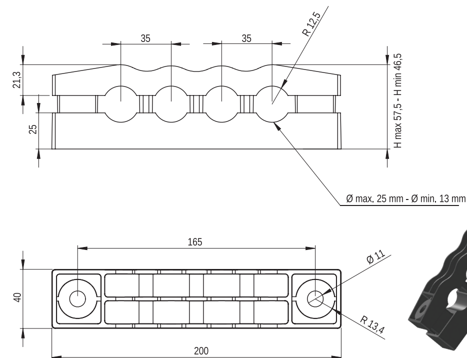
Obejma kablowa KO 4/13-25
