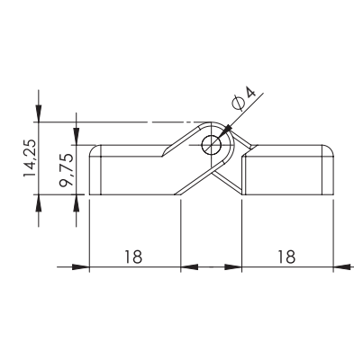
Zawias ZM48N
