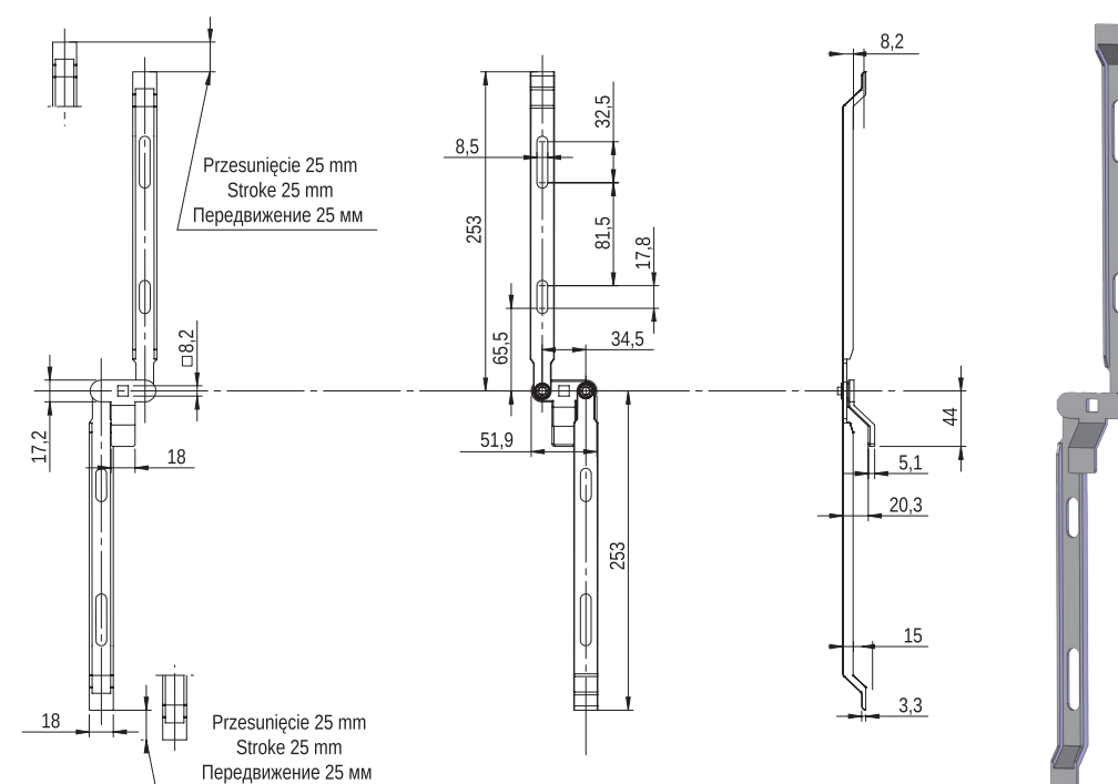
Сігна з механізмом obrotowym Cmo2
