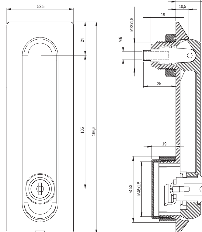
Zamek HS 08N
