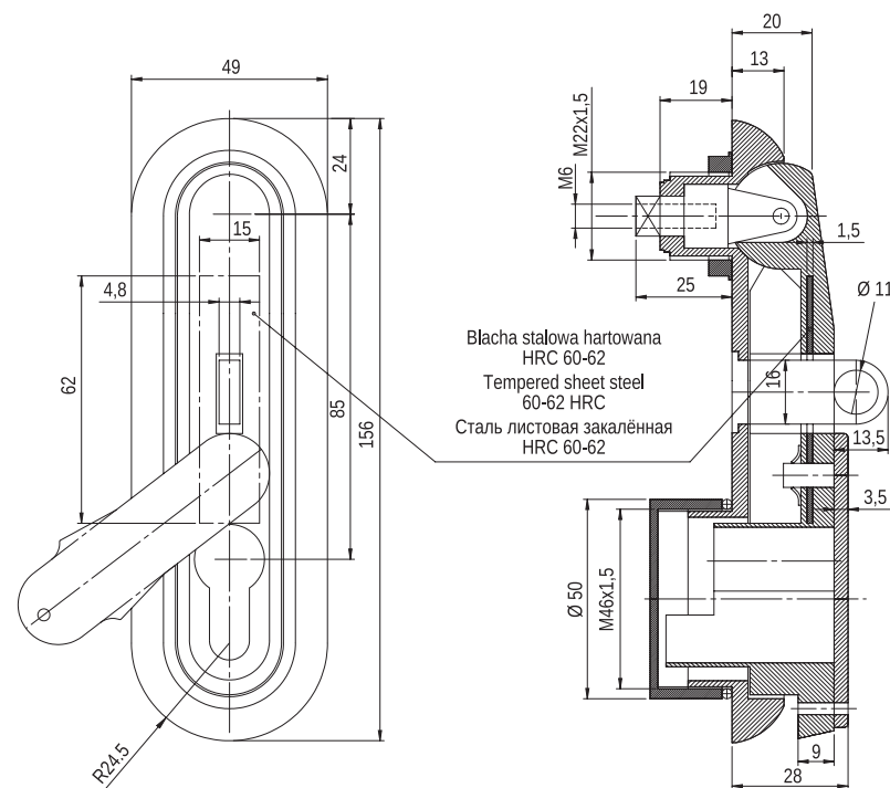
Zamek HS 06/B
