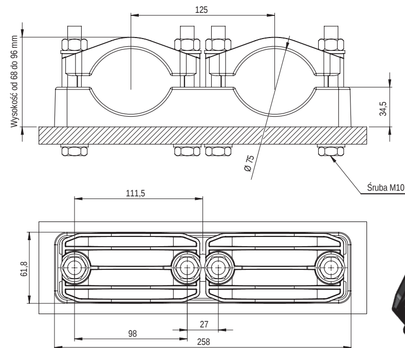
Obejma kablowa zespolona KO 75/2
