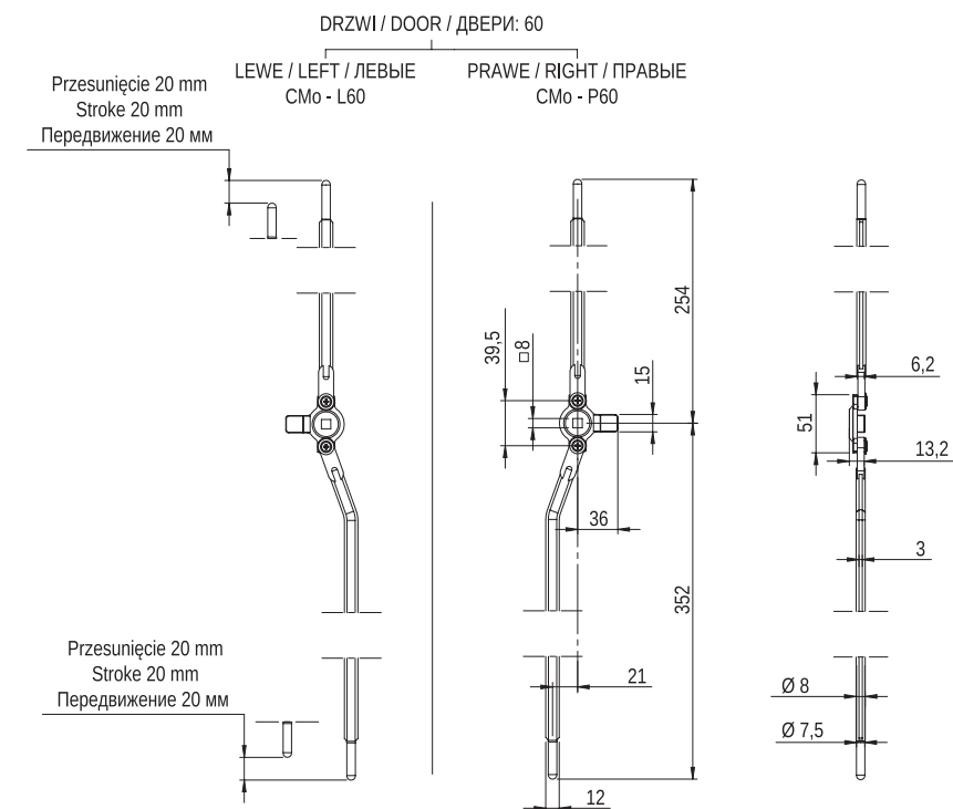
Cięgna z mechanizmem obrotowym Cmo - P, L 60
