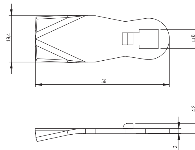
Język do zamka HS na mechanizm zębata - wersja prosta
