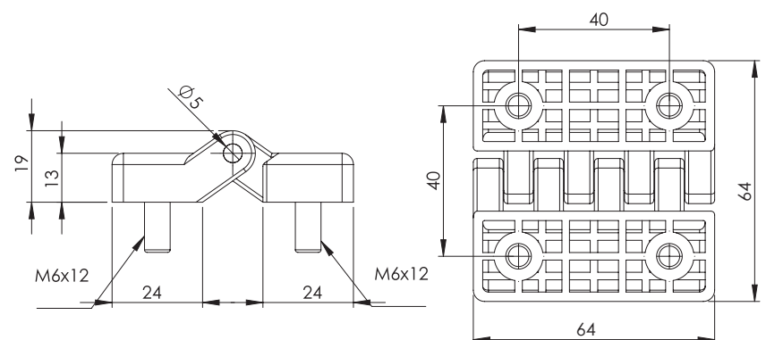
Zawias ZM64S
