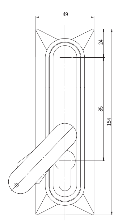
Zamek HS 01 prostokątny MATERIAL: Korpus - PA 6 GF30; kolor czarny, biały, szary wg RAL.
