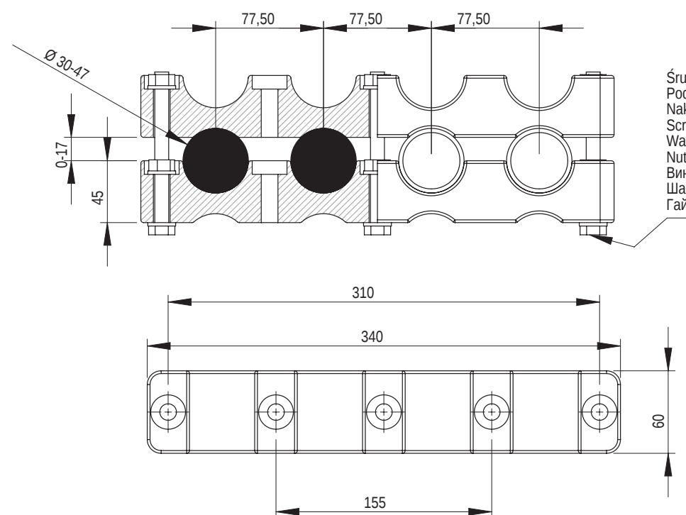
Obejma kablowa zespolona KO 4 30-47
