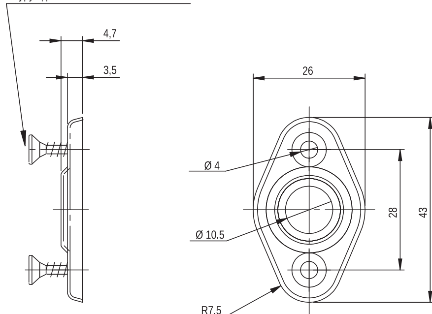
Szyld zamka typu B z
