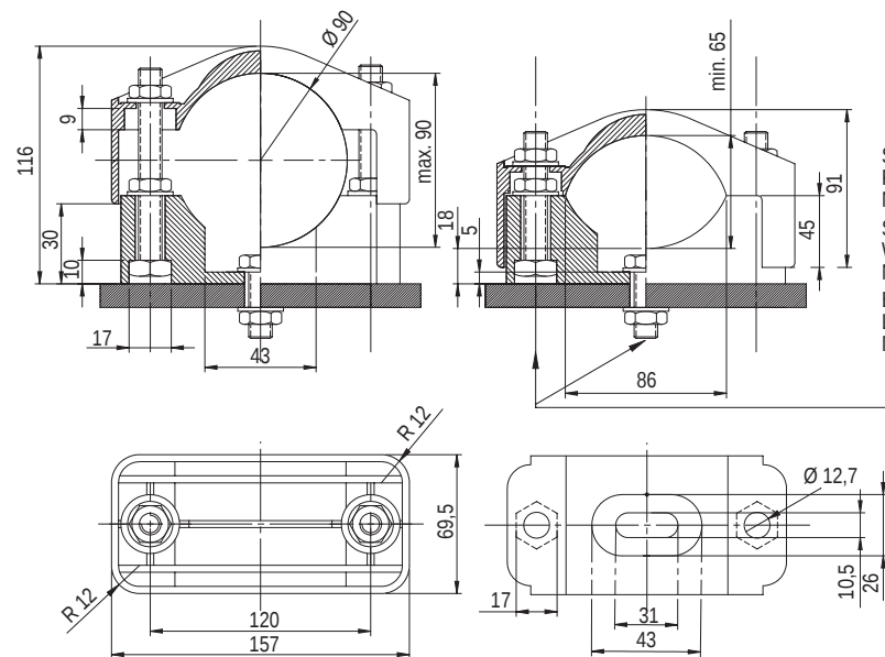
Obejma kablowa KO 90
