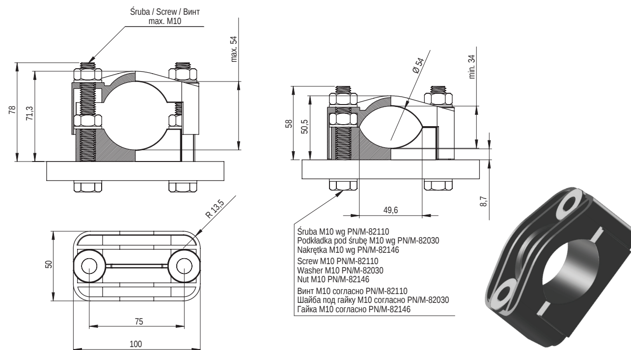
Obejma kablowa KO 54
