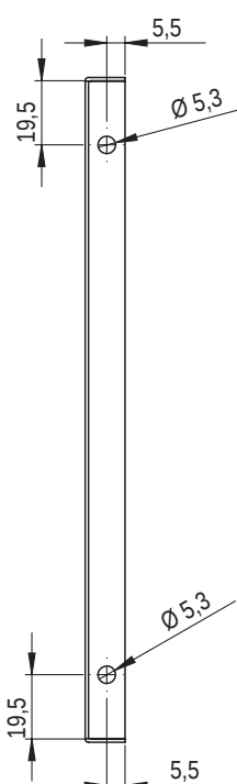
Rozmieszczenie otworów montażowych
