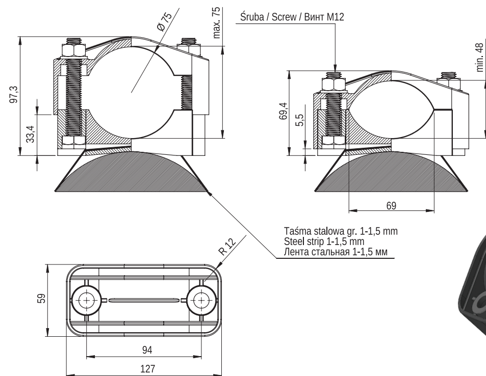
Obejma kablowa KO 75 TO
