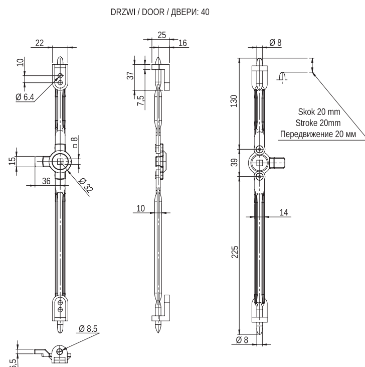
Сігна з механізмом obrotowym Cmo1 - P, L 40
