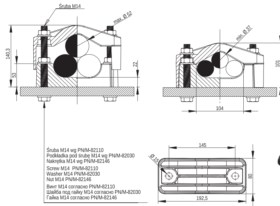
Obejma kablowa KO 3 37-52
