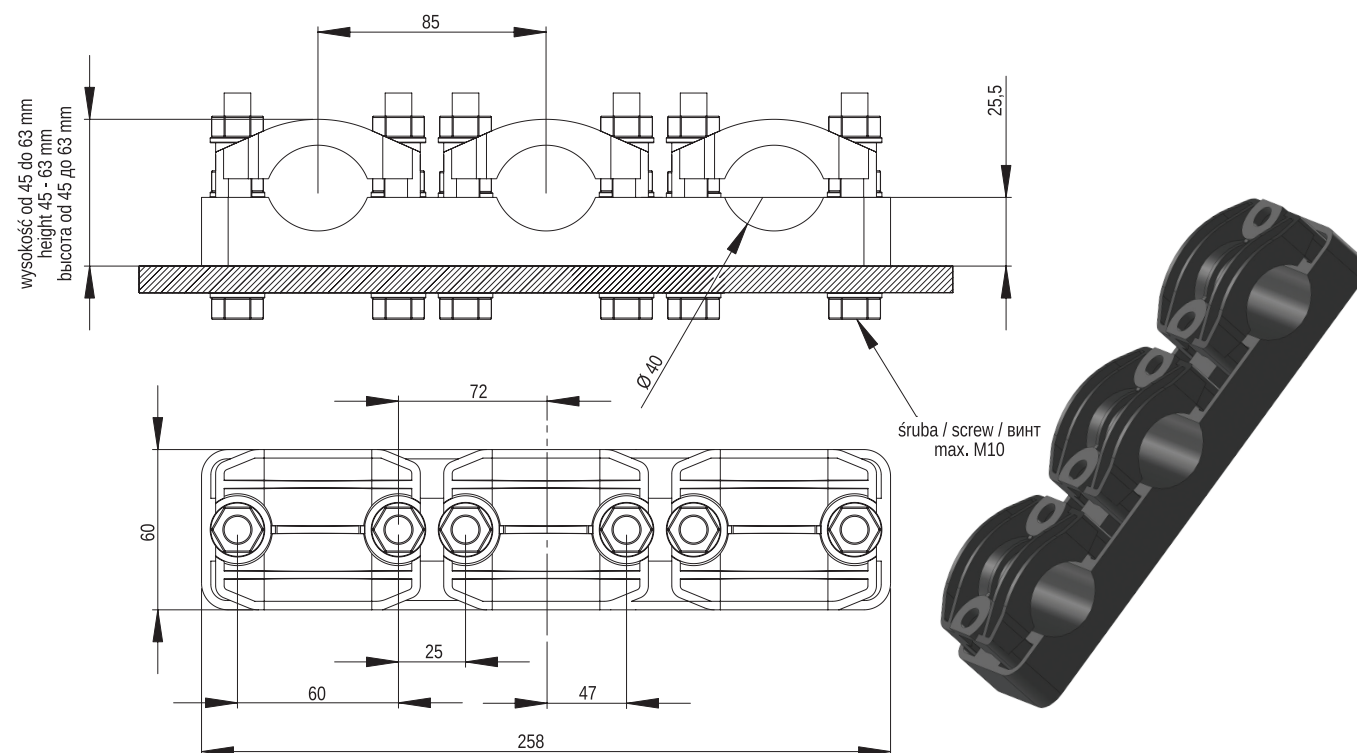
Obejma kablowa zespolona KO 40/3
