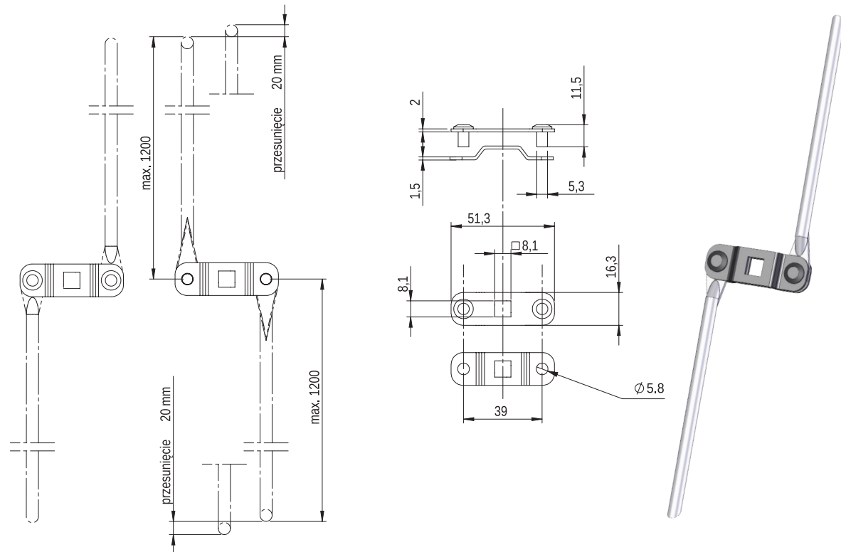
Blaszki do cięgien metalowych 'kwadrat'
