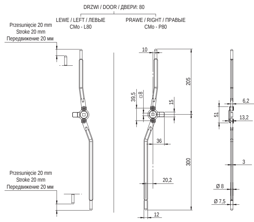
Сігна з механізмом обrotowym Cmo - P, L 80
