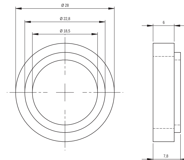
Podwyższenie prowadnicy PR6/2 i PR8/2
