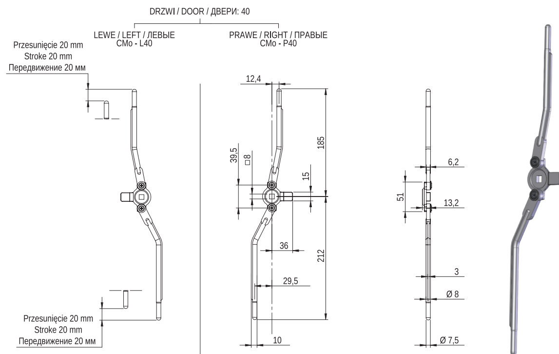
Cięgna z mechanizmem obrotowym Cmo - P, L 40
