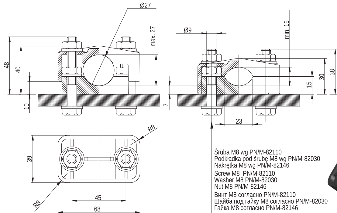
Obejma kablowa KO 27
