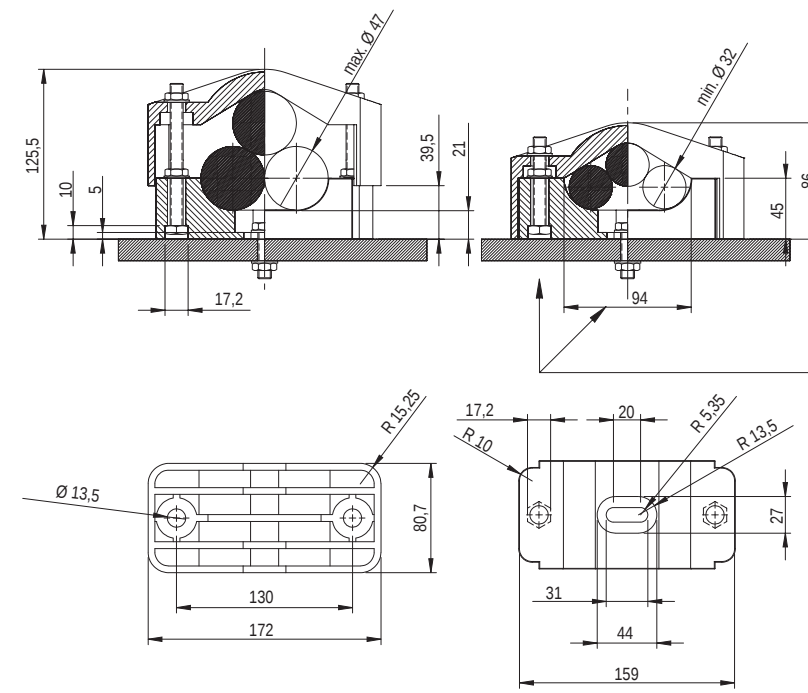
Obejma kablowa KO 3 32-47
