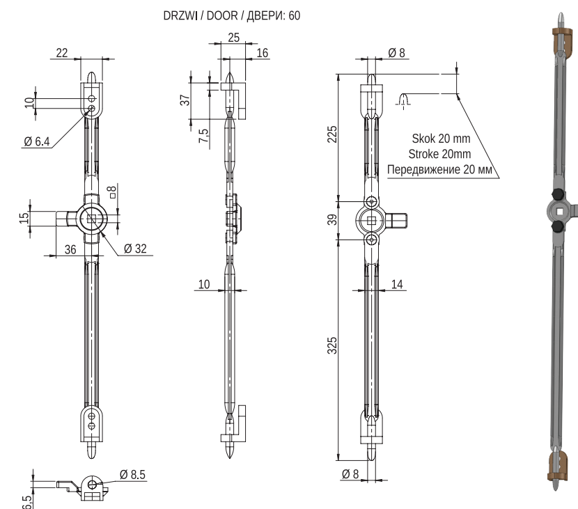
Сігна з механізмом obrotowym Cmo1 - P, L 60
