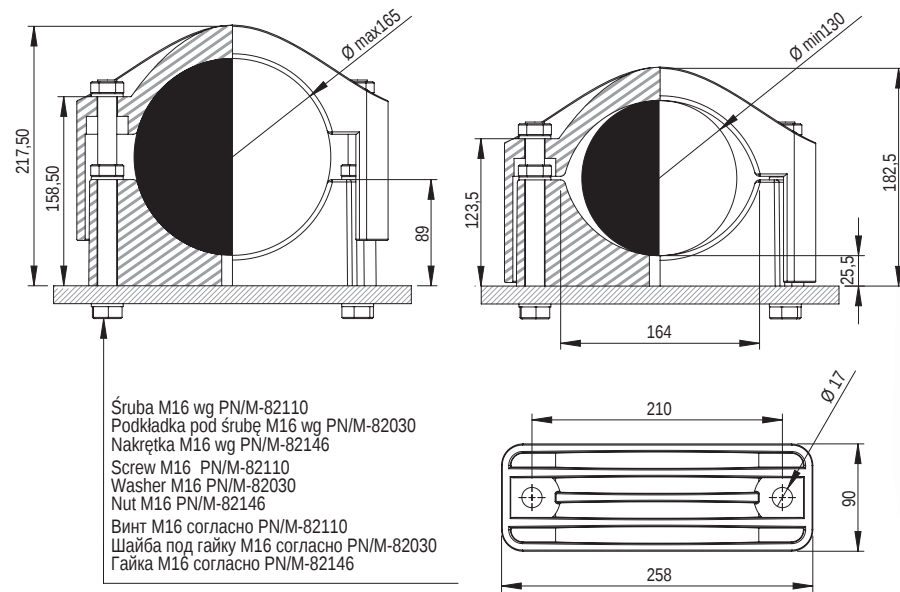
Obejma kablowa KO 165
